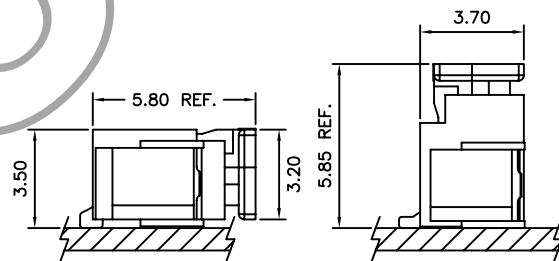
SMT TYPE
