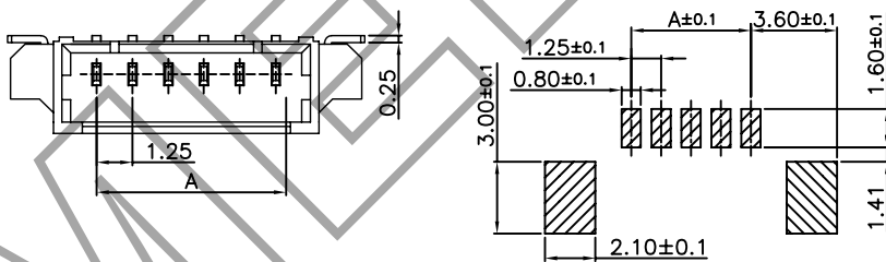
P.C.B LAYOUT
